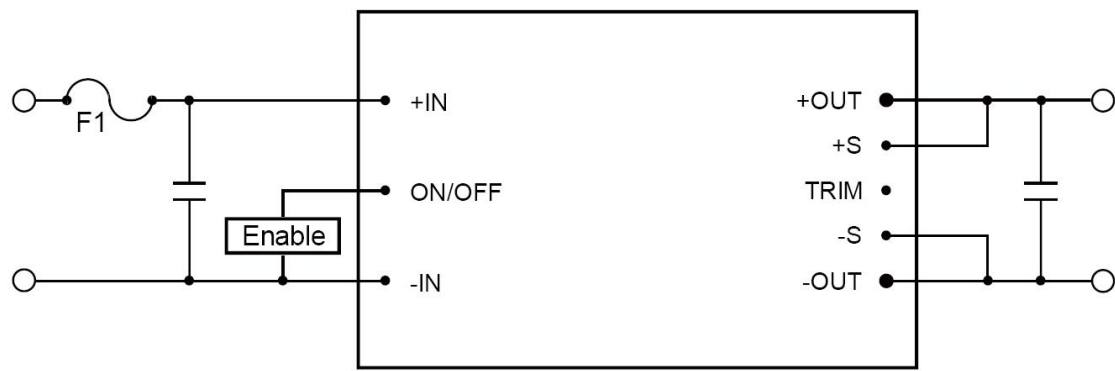
模块运行示意图
