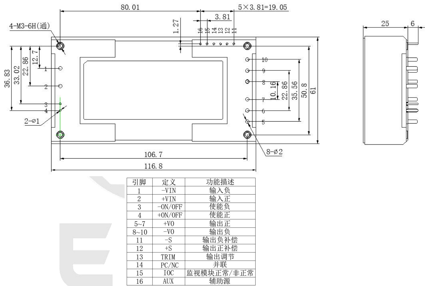
图2：产品外观示意图
